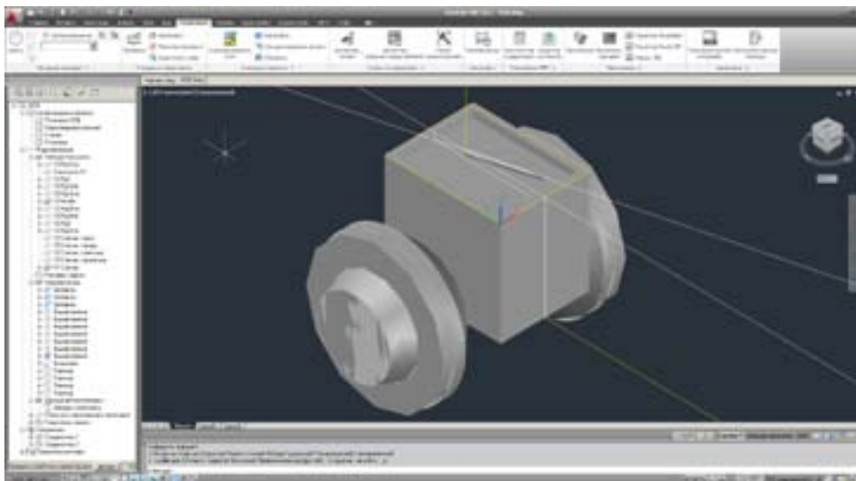
Параметрическая модель ротаметра, выполненная в AutoCAD MEP
