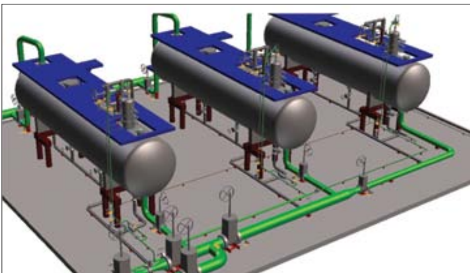
Модель установки подготовки пластовой воды, выполненная в AutoCAD MEP
