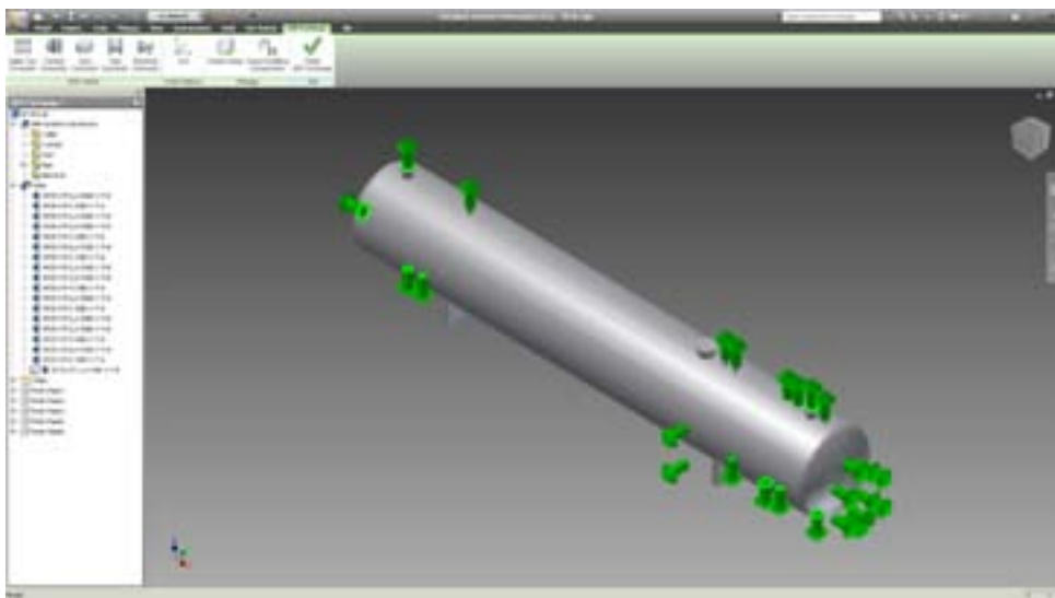
Параметрическая модель сепаратора НГСВ, выполненная в Inventor и подготовленная для экспорта в AutoCAD MEP
